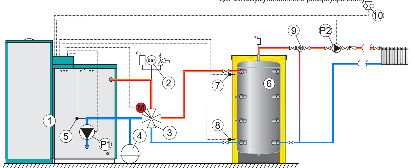
Схема 6. Конфигурация AKU -- IKG (аккумуляция - не прямой круг отопления)
