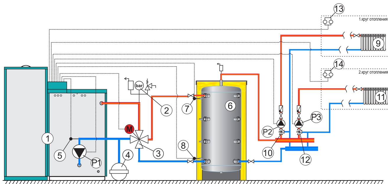
Схема 14. Конфигурация AKU--IKGX2
