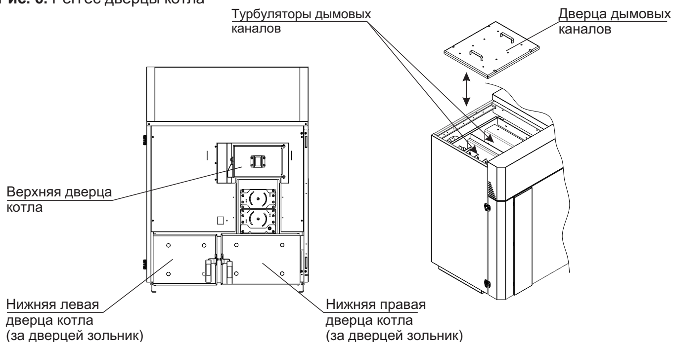
Рис. 6. PelTec дверцы котла
