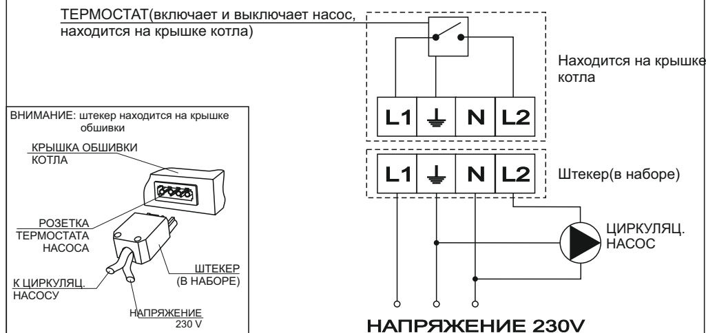
Схема 4. Электрическая схема подключения для топки твердым топливом
