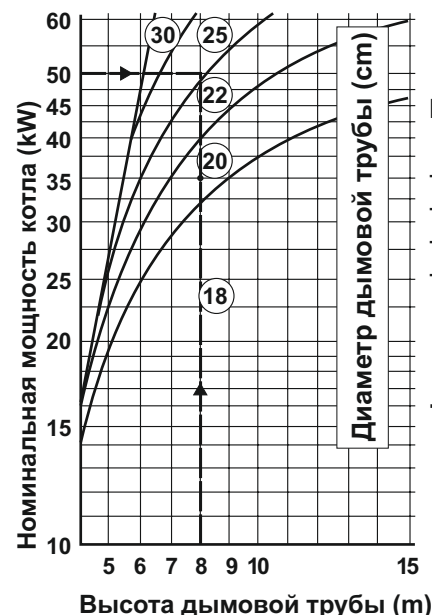
Рис 4. Размеры дымовой трубы для котла CentroPlus
