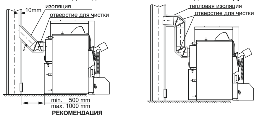
Рис 3. Возможный вид соединения котла CentroPlus к дымовой трубе
