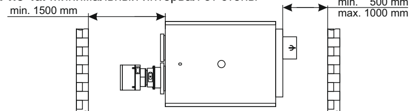
Рис 4а. Минимальный интервал от стены
