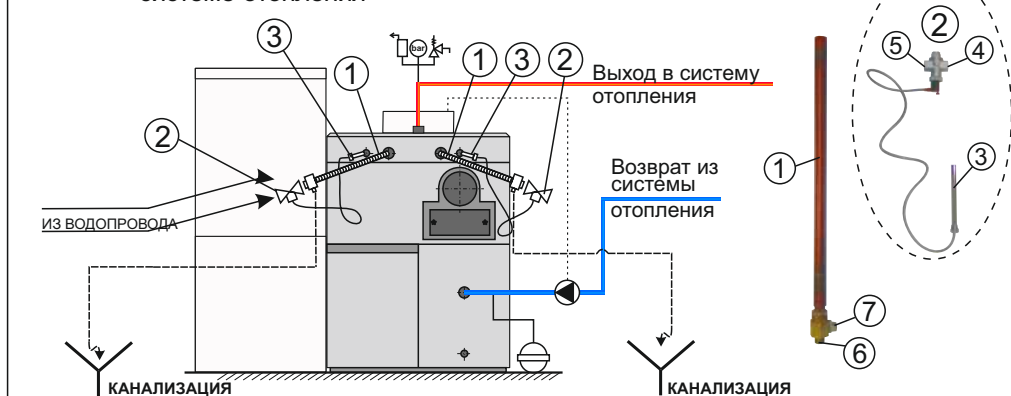
Схема 2.1. Монтаж термической защиты котла CentroPlus 50 при закрытой системе отопления
