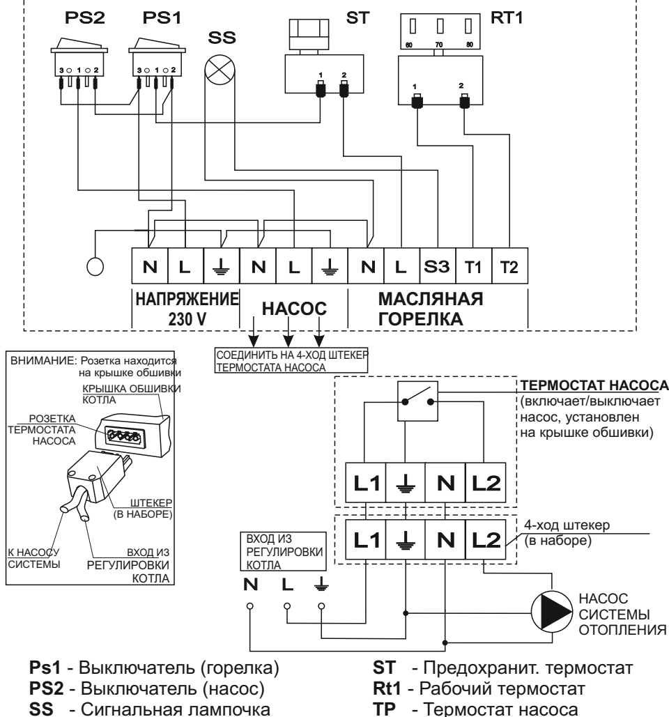
Схема 5. Электрическая схема регулировки котла ЕКО СК/СКВ на твердое/жидкое топливо и термостата насоса
