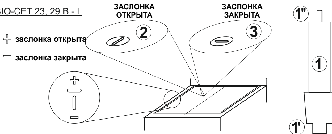
Рис. 3. Использование заслонки для растопки котла
