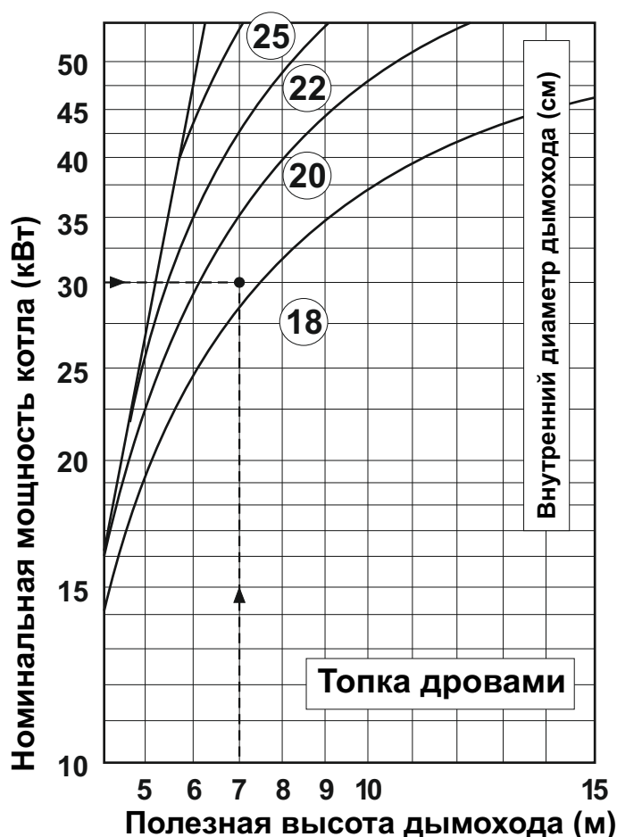
Рис. 1. Размеры дымохода для BIO-CET 23, 29 В
