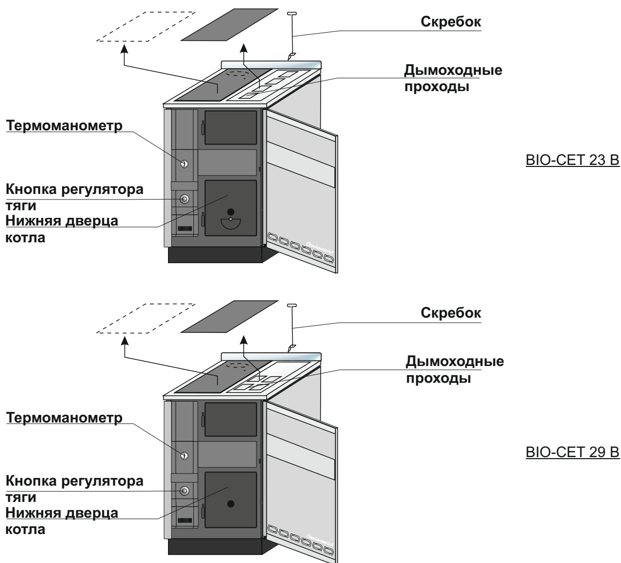
Рис. 7. Очистка поверхностей - BIO-CET B-L(верно и для котла BIO-CET B - D)
