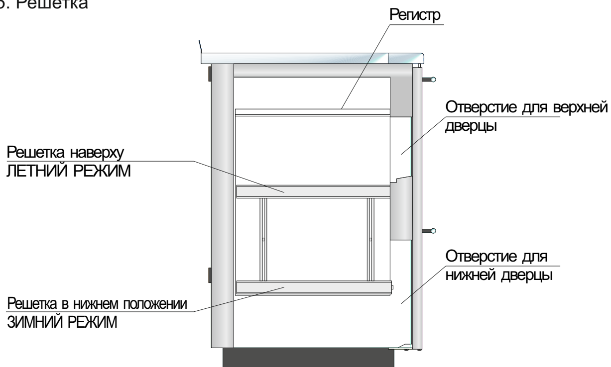
Рис. 5. Решетка
