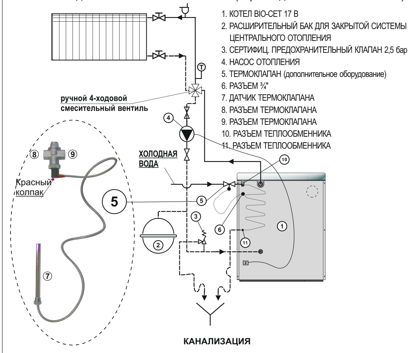
Схема 2. - Подключение котла BIO-CET В - L (верно и для котла BIO-CET В - D)
