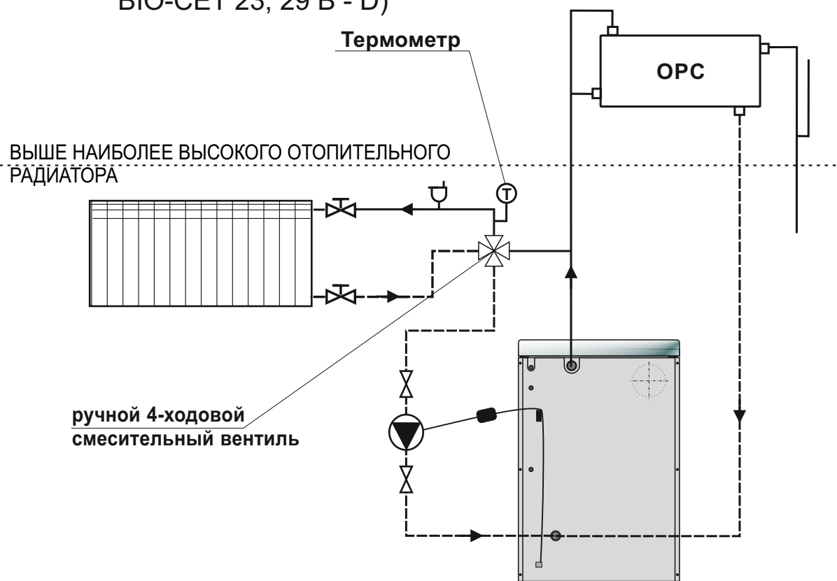
Схема 1. Подключение котла - BIO-CET 23, 29 В - L (верно и для котла BIO-CET 23, 29 В - D)
